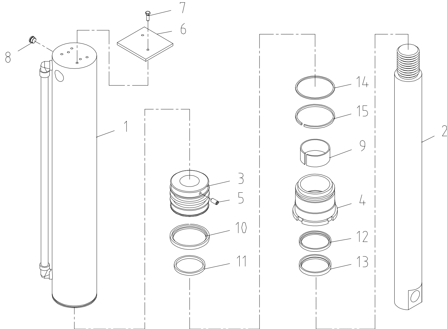
잭 실린더 조립체 Fig. 4-2 SCS1015LSuper JACK CYL' ASS'Y
