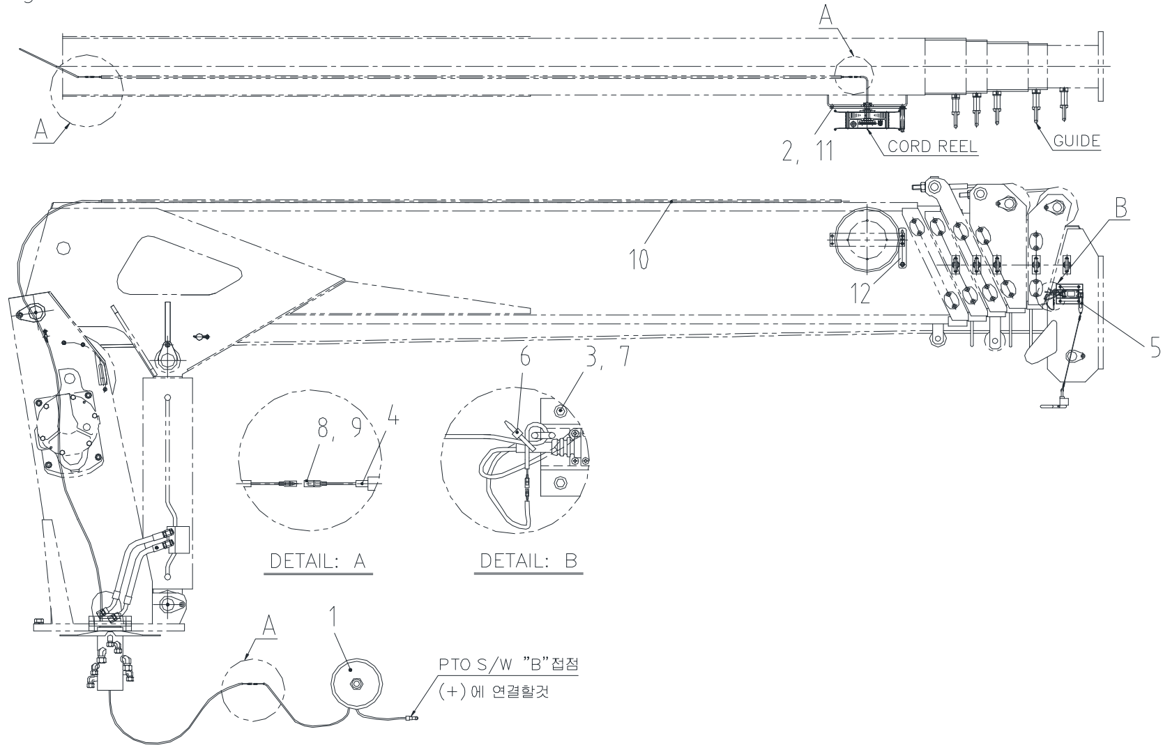
Fig. 15 과권방지장치 조립체
