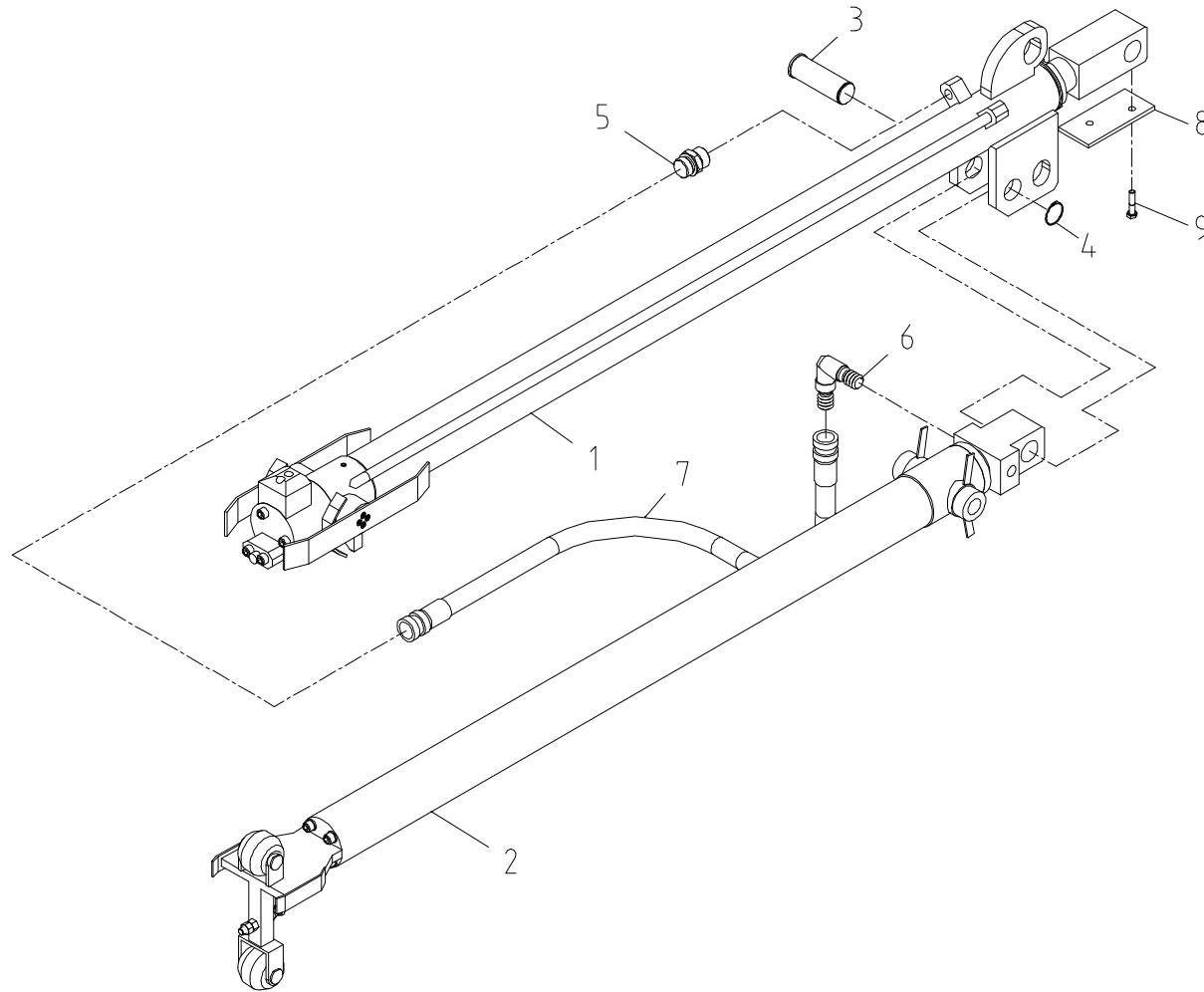
텔레스코픽 실린더 조립체 Fig. 1-1 SCS1015LSuper TELESCOPIC CYLINDER ASS'Y
