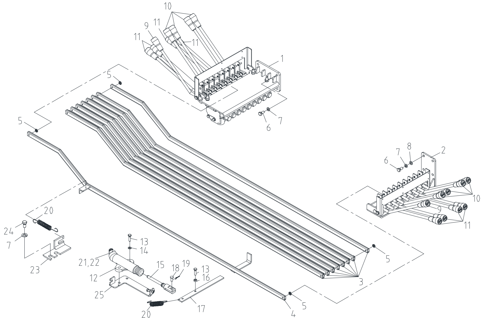
오퍼레이션 조립체 Fig. 3-2 SCS1015LSuper OPERATION ASS'Y
