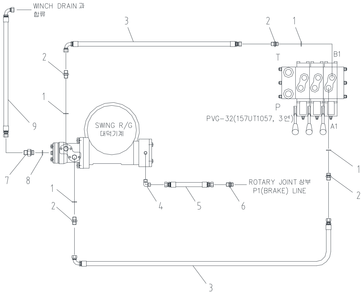
스윙 배관 Fig. 5-2 SCS1015LSuper SWING PIPING
