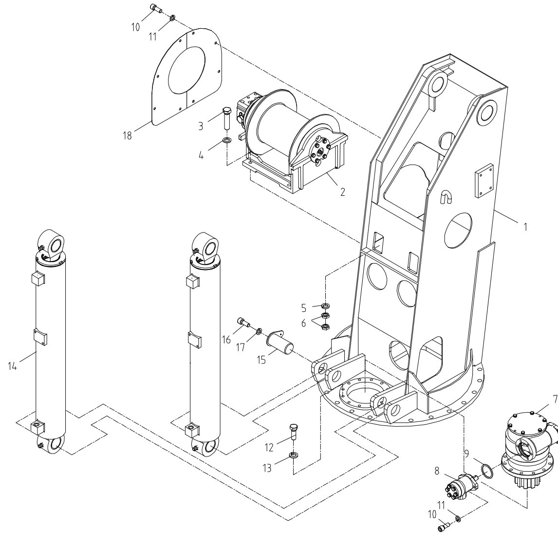
스윙 포스트 조립체 Fig. 2 SCS1015LSuper SWING POST ASS'Y
