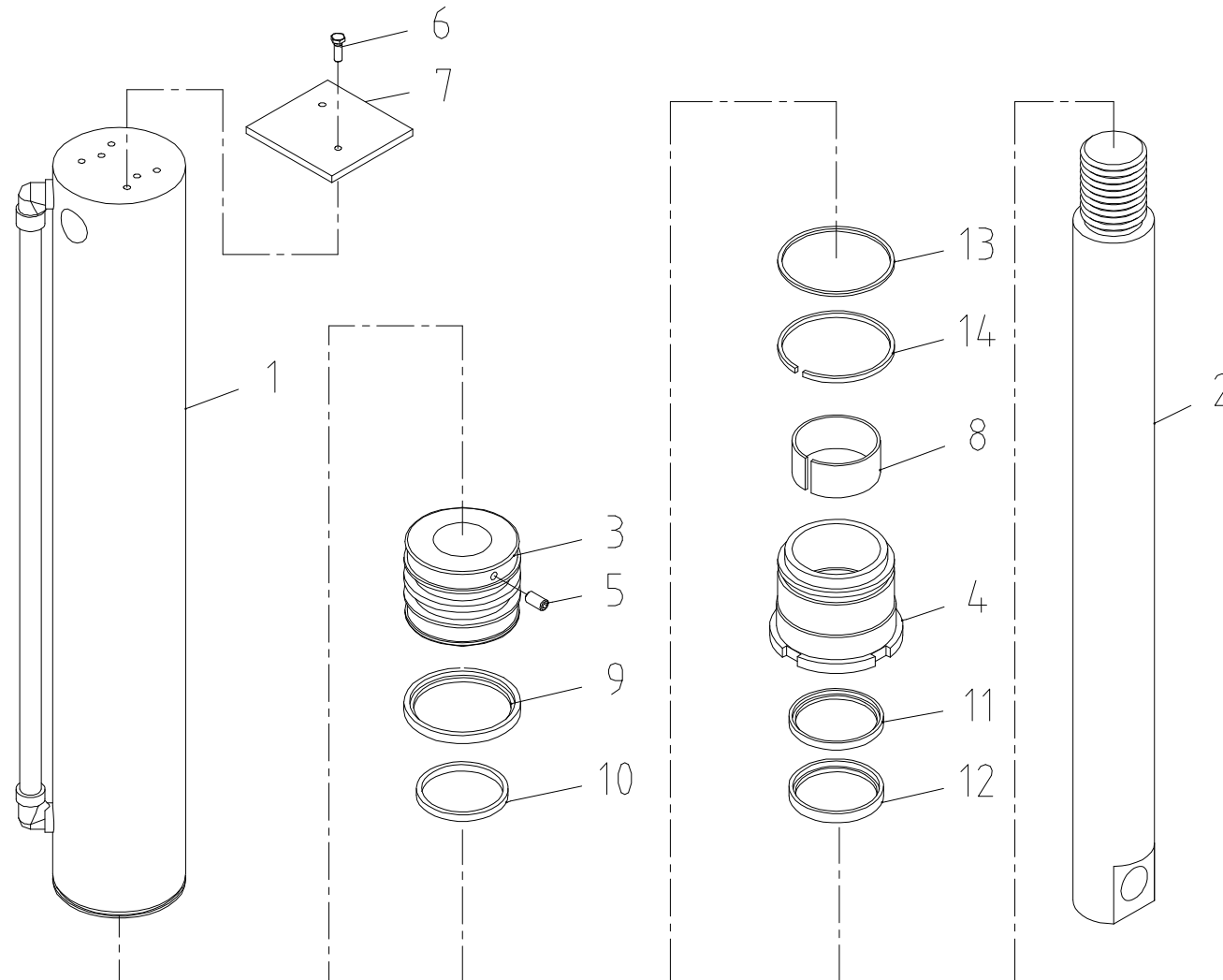
잭 실린더 조립체 Fig. 10-2-1-1 SCS1015LSuper JACK CYL' ASS'Y
