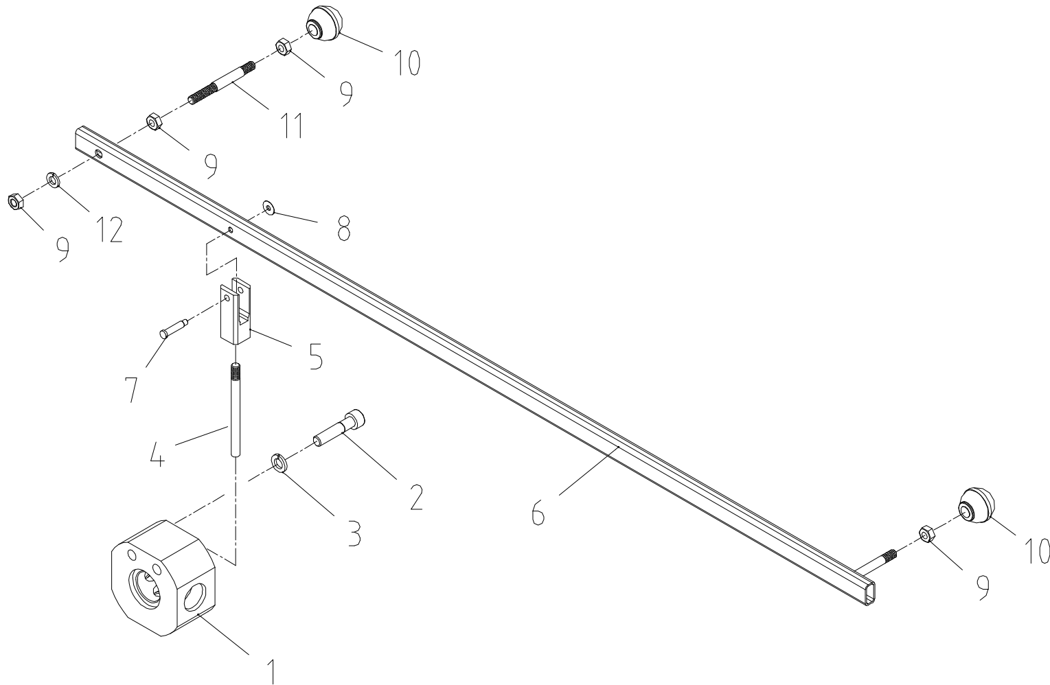
디버터 밸브 셋트 Fig. 3-3 SCS1015LSuper DIVERTER V/V SET
