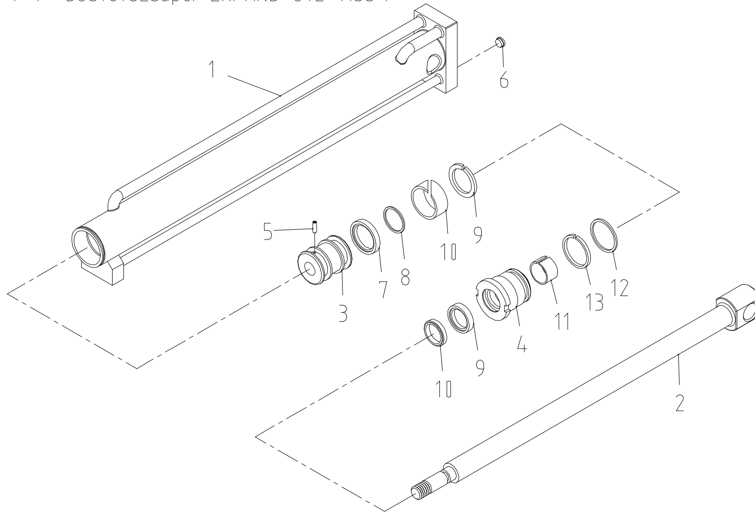
익스펜드 실린더 조립체 Fig. 4-1 SCS1015LSuper EXPAND CYL' ASS'Y
