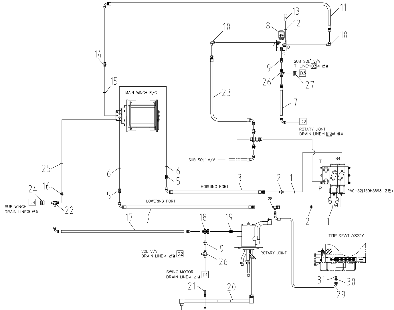
메인 윈치 배관 Fig. 5-5 SCS1015LSuper MAIN WINCH PIPING
