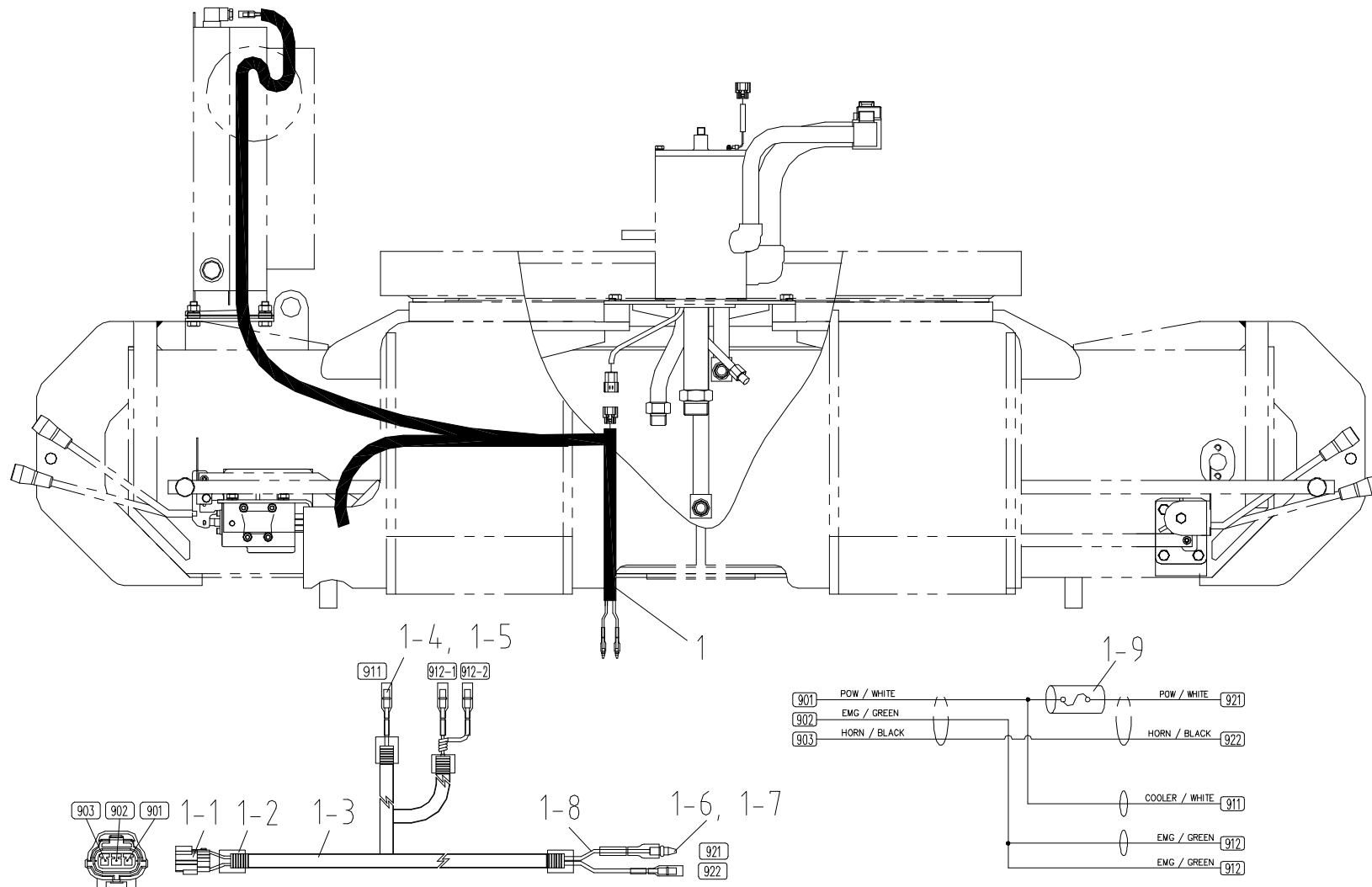
프레임 전선 Fig. 11-1. SCS1015LS FRAME WIRING
