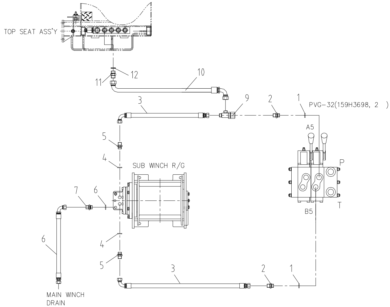
보조 윈치 배관 Fig. 14 SUB WINCH PIPING
