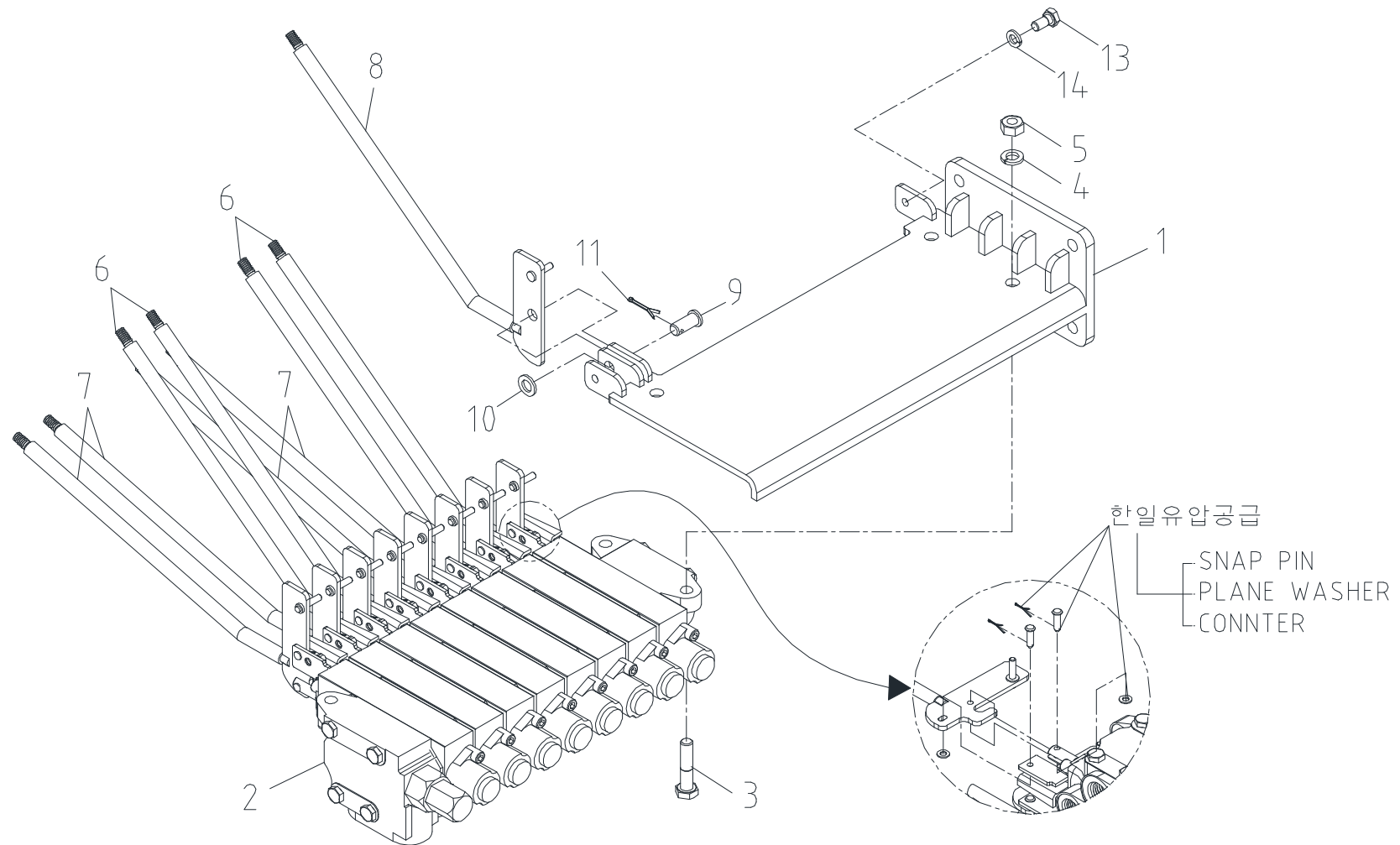
밸브 스텐드 셋 Fig. 3-2-1 SCS1015LSuper VALVE STAND SET
