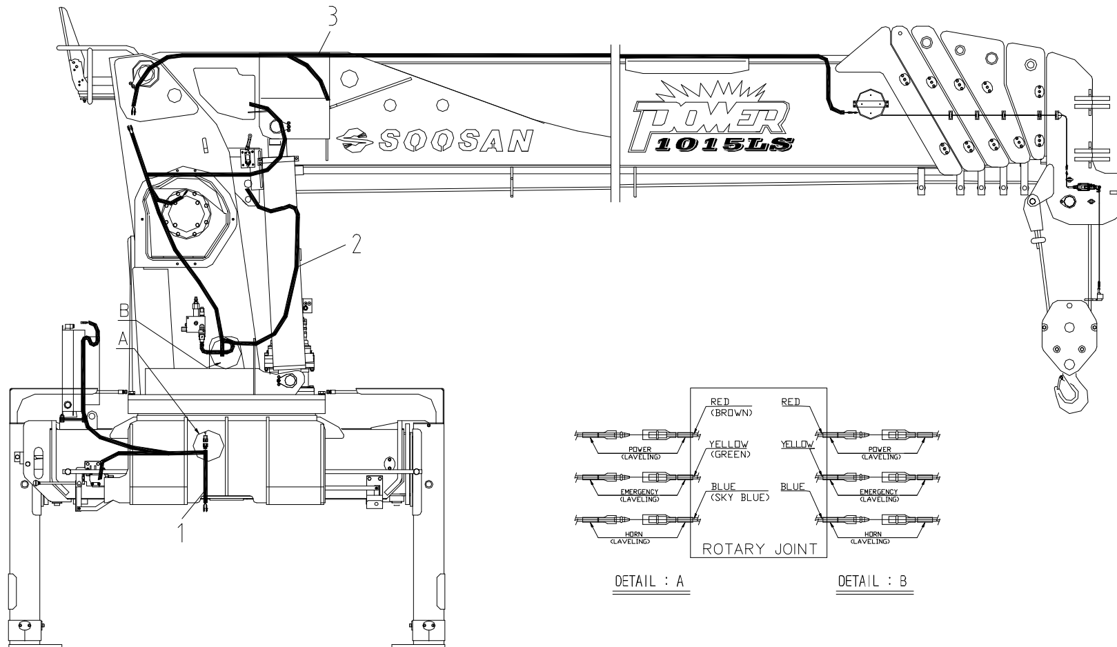
전선 조립체 Fig. 11 SCS1015LS WIRING ASS'Y
