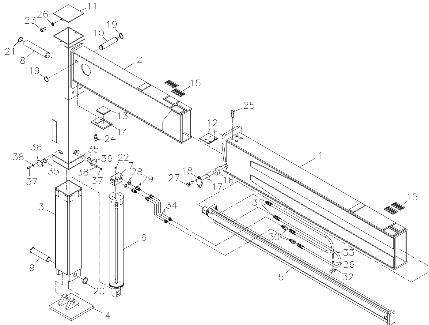
아우트리거 조립체 Fig. 4 SCS1015LSuper OUTRIGGER ASS'Y
